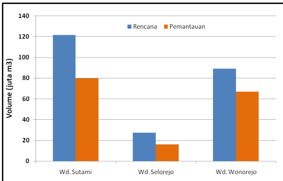
Gambar 5. Perbandingan Volume Rencana dan Pemantauan 3 Waduk Utama di Jawa Timur (Status 01 s/d 15 September 2019)
