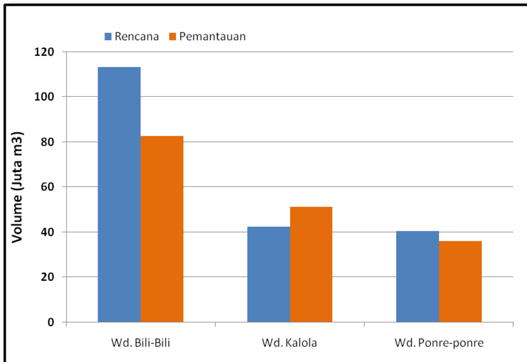
Gambar 6. Perbandingan Volume Rencana dan Pemantauan 3 Waduk Utama di Sulawesi Selatan (Status 01 s/d 15 September 2019)
