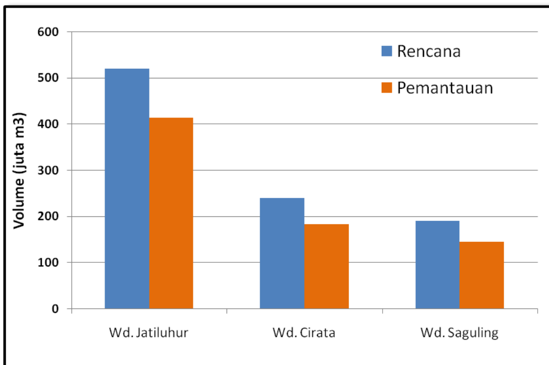
Gambar 3. Perbandingan Volume Rencana dan Pemantauan 3 Waduk Utama di Jawa Barat (Status 01 s/d 15 September 2019)
