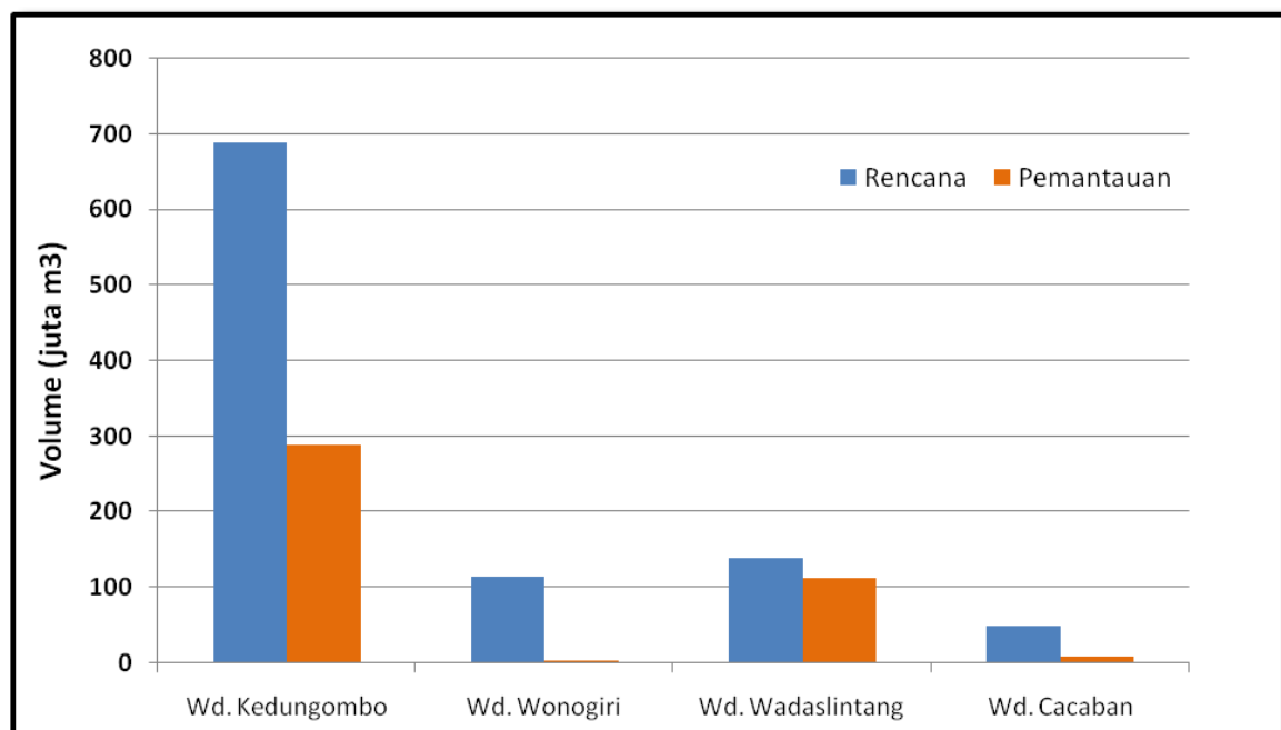
Gambar 4. Perbandingan Volume Rencana dan Pemantauan 4 Waduk Utama di Jawa Tengah (Status 01 s/d 15 September 2019)
